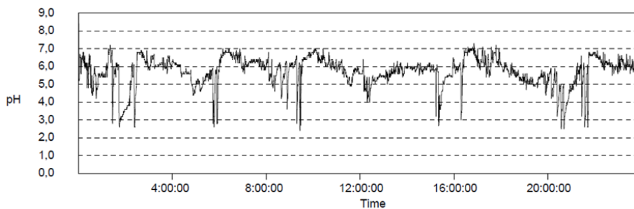
Voorbeeld van curve met resultaat van pH-metrie
